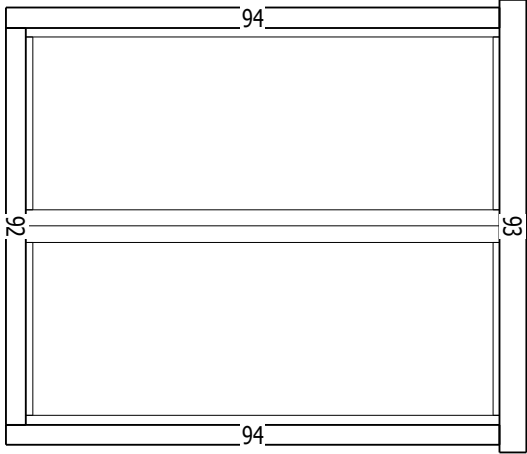
DOUBLE DOOR 1615X1920
