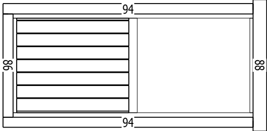
DOOR 850X1920
